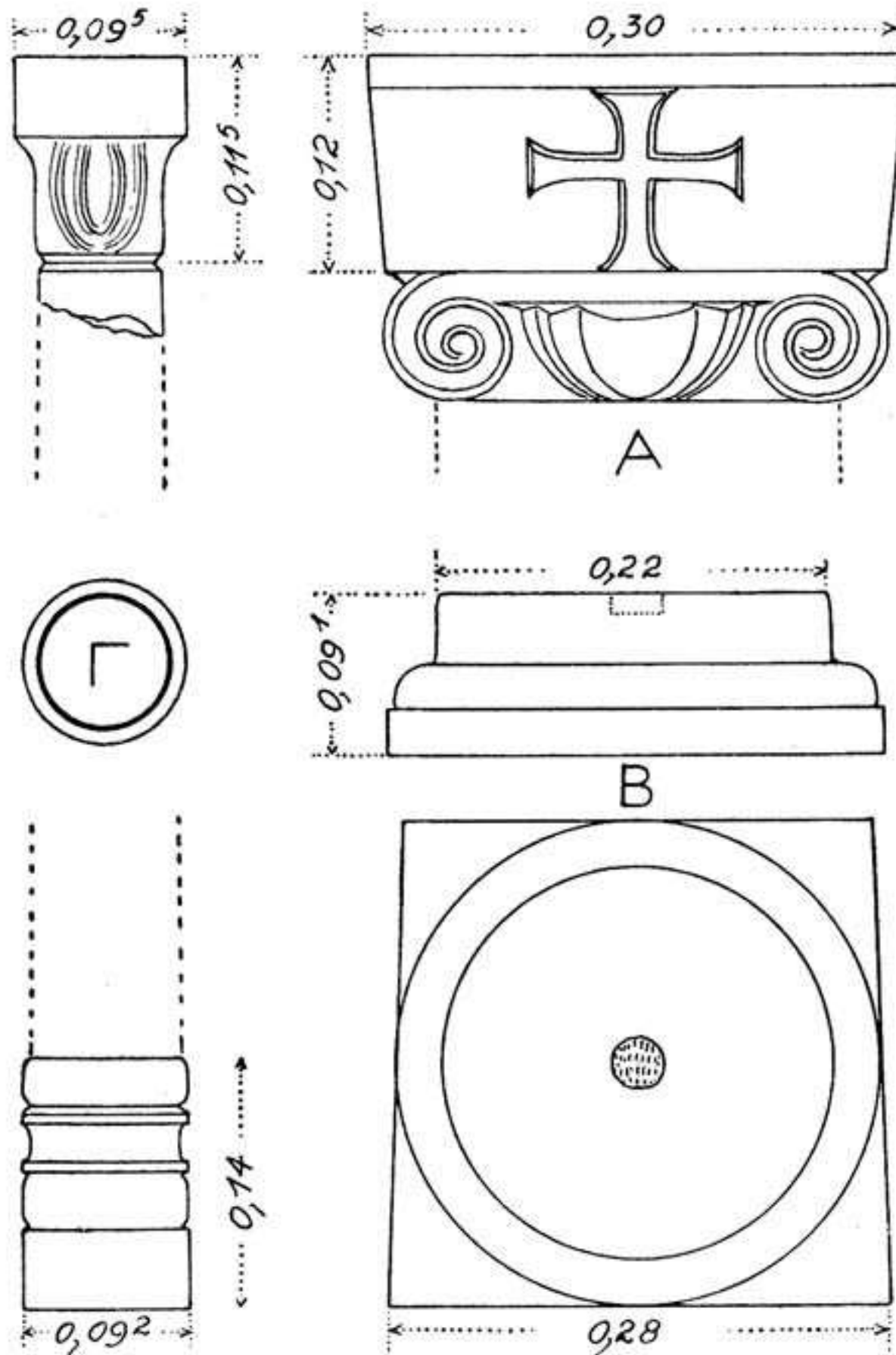
Εἰκ. 5.—Κιονόκρανον τῶν κίωνων τῶν κιονοστοιχιῶν (ἄνω ἀριστερᾷ), βᾶσις τοῦ κιβωρίου (κάτω δεξιᾷ) καὶ κιονίσκος τῆς Ἀγ. Τραπεζῆς (ἀριστερᾷ).
