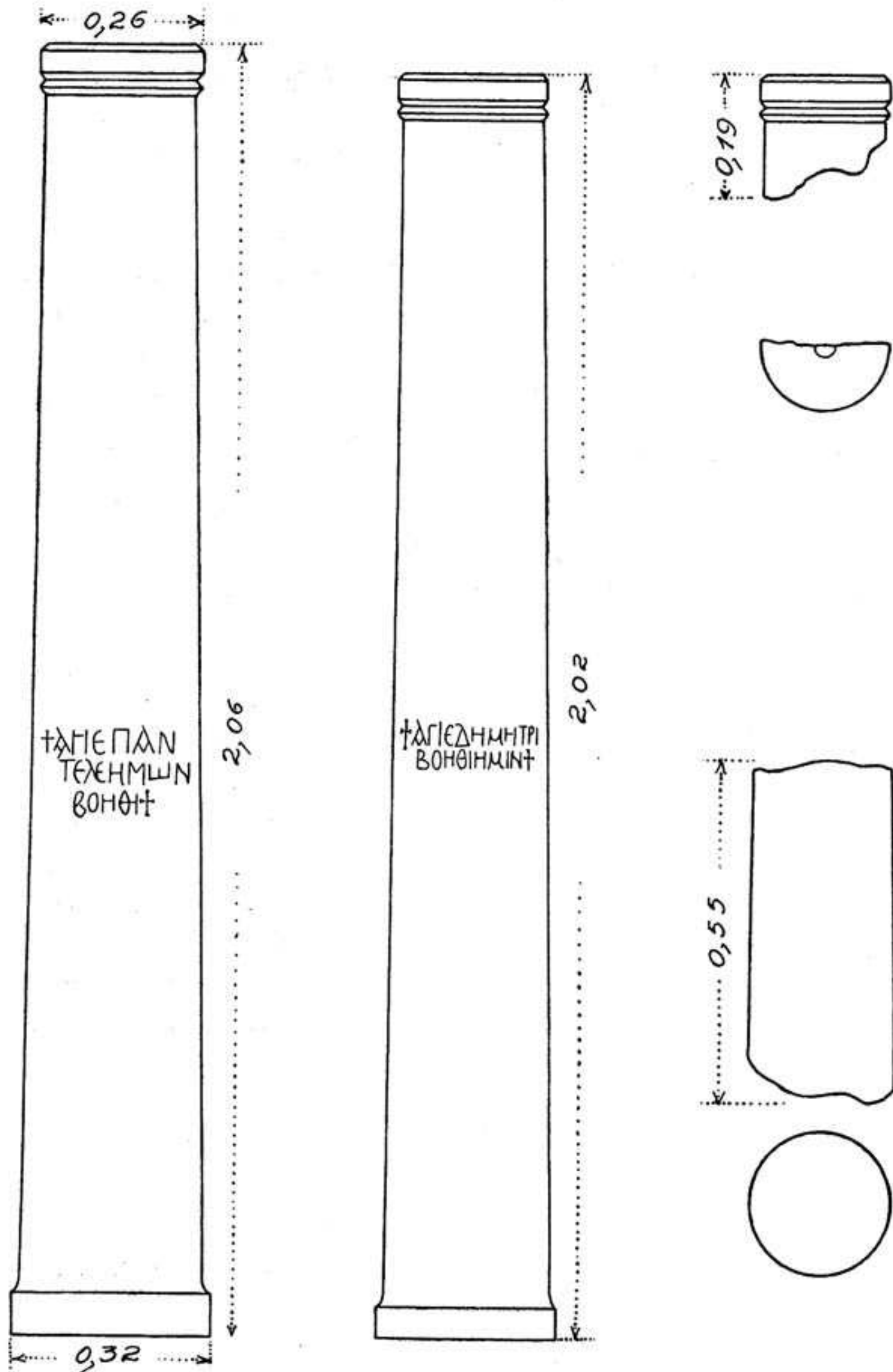
Εἰκ. 3.—Οἱ διασωθέντες κορμοὶ κίωνων τῶν ἐσωτερικῶν κιονοστοιχιῶν τῆς βασιλικῆς.
