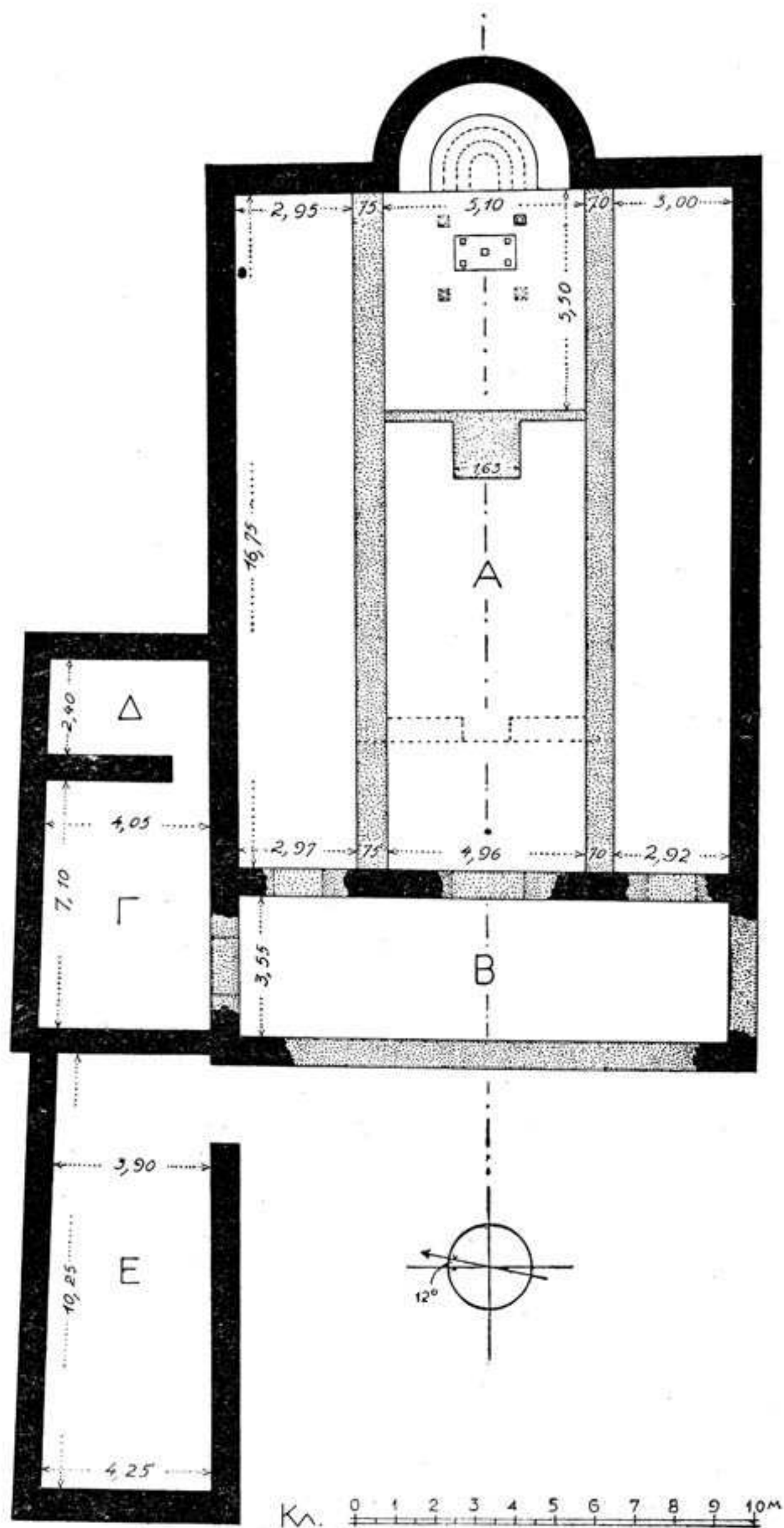
Εἰκ. 2.—Γενικὴ κάτοψις τῆς βασιλικῆς τῆς Σινίας.
